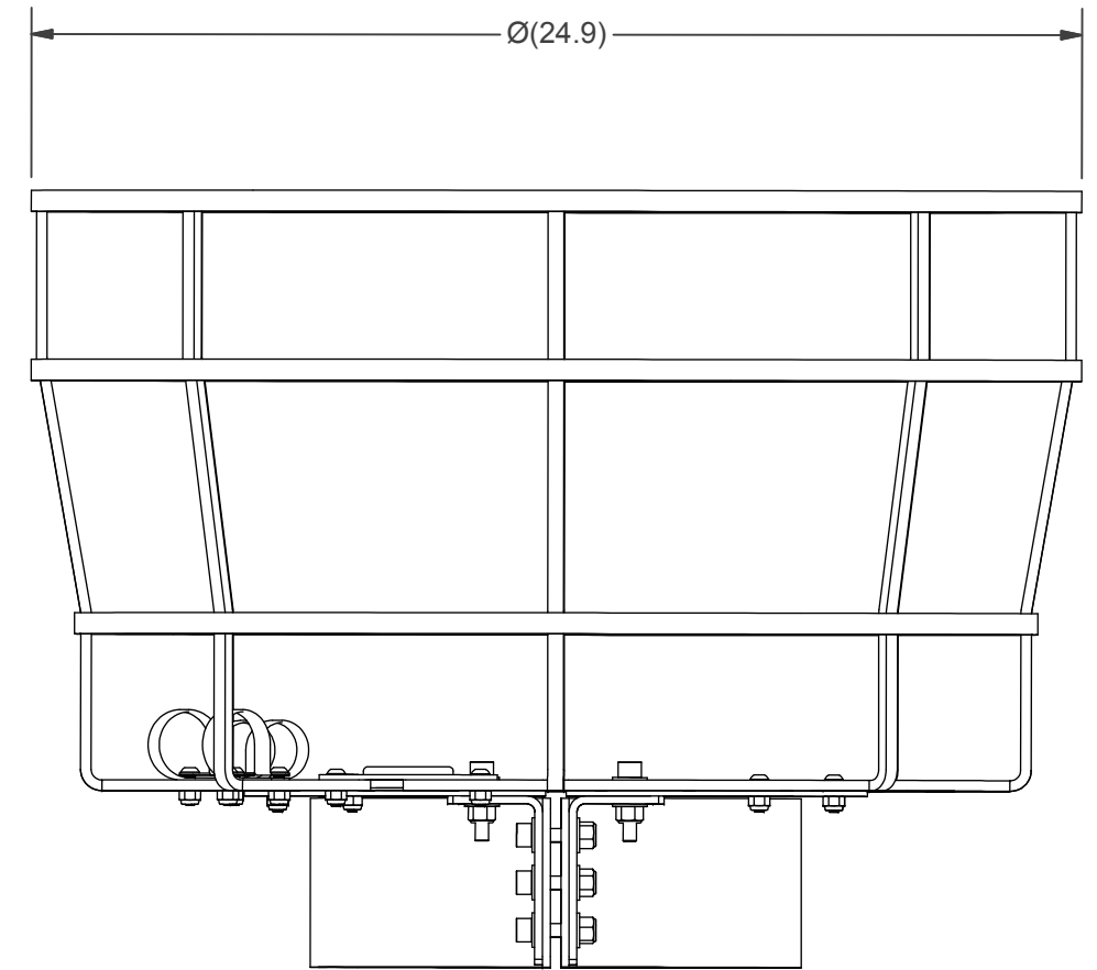
VIEW A-A
